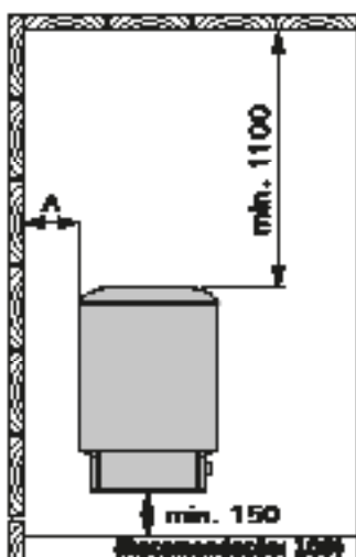
Tabulka 2. Podrobnosti montáže topného tělesa
