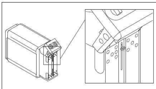
Figure 7. Connecting the connection cable Abbildung 7. Befestigung des Anschlusskabels
