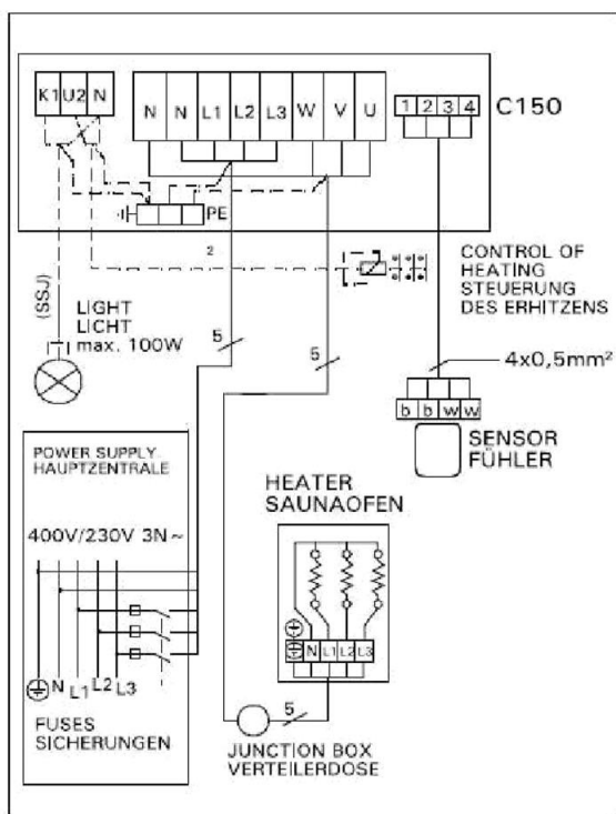
Obrázek 13: Elektrické připojení kontrolní jednotky C90/C150 a ohřivače ME
