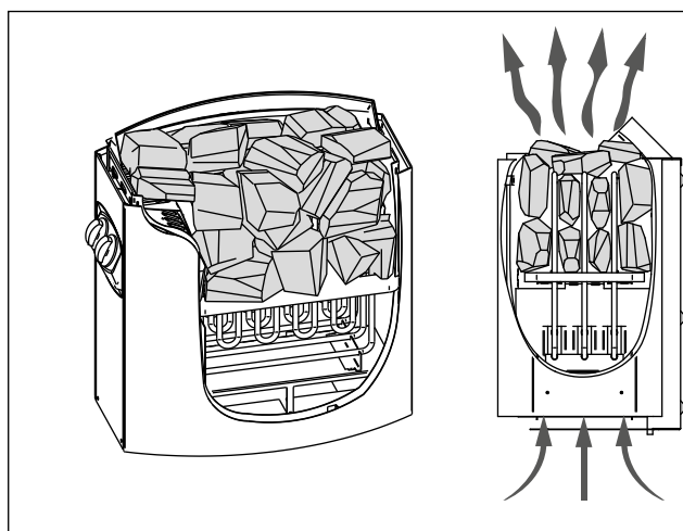
Rys. 1. Układanie kamieni w piecu Obr. 1. Skládání topných kamenů
