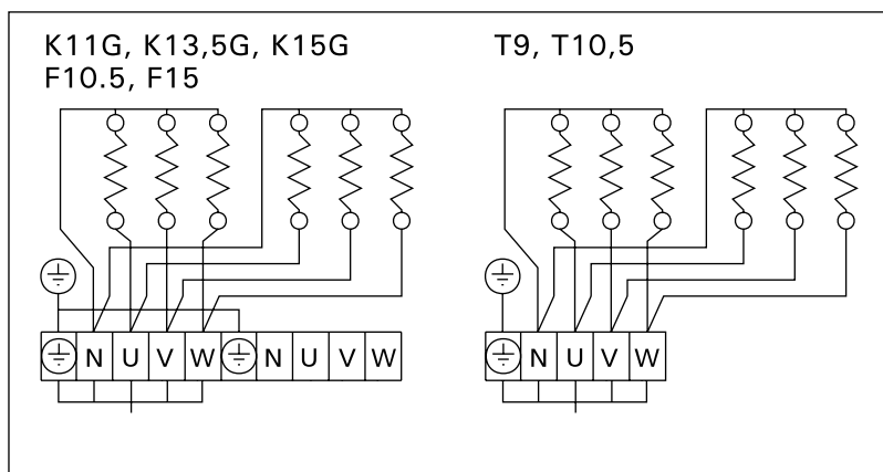
Rys. 5. Przyłącza elektryczne pieca Obrázek 5. Zapojení topného tělesa
