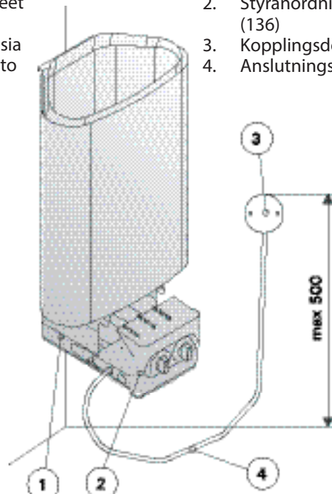
Kuva 9. Kiukaan kytkentä Bild 9. Anslutning av aggregat
