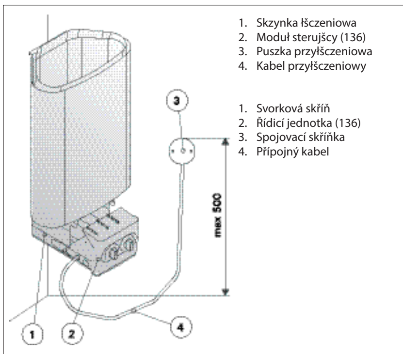
Rys. 9. Podláščení elektryczne grzejnika Obrázek 9. Připojky kamen
