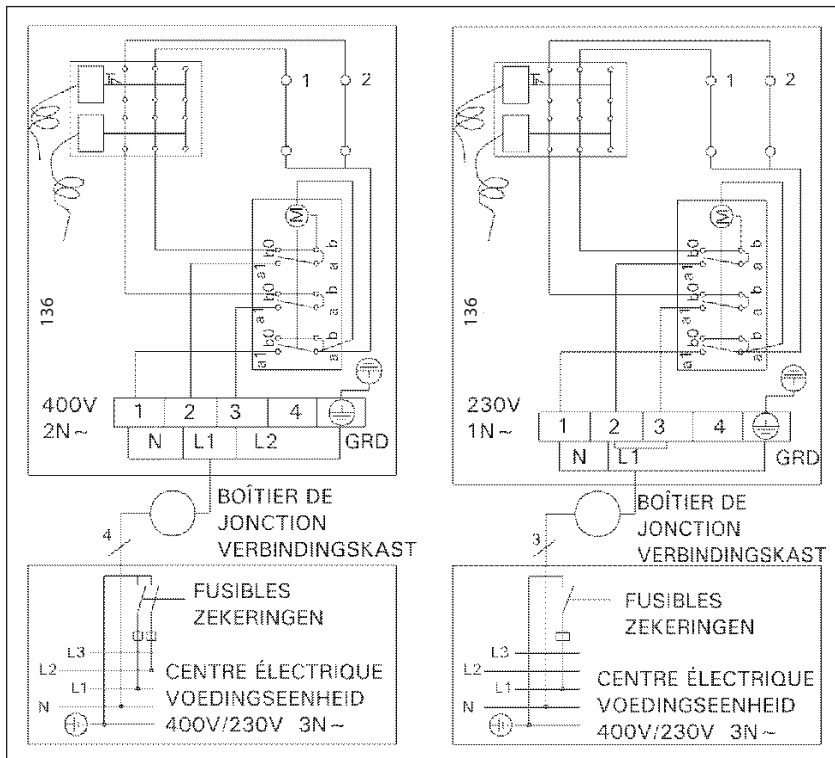
Figure 10. Raccords électriques du pôle (136) Figuur 10. Elektrische aansluitingen van de saunaoven (136)
