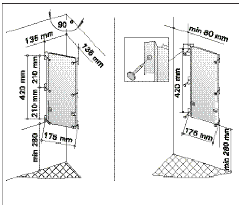
Figure 7. Location of the mounting rack of the heater Abbildung 7. Platz des Montagegestells des Saunaofens
