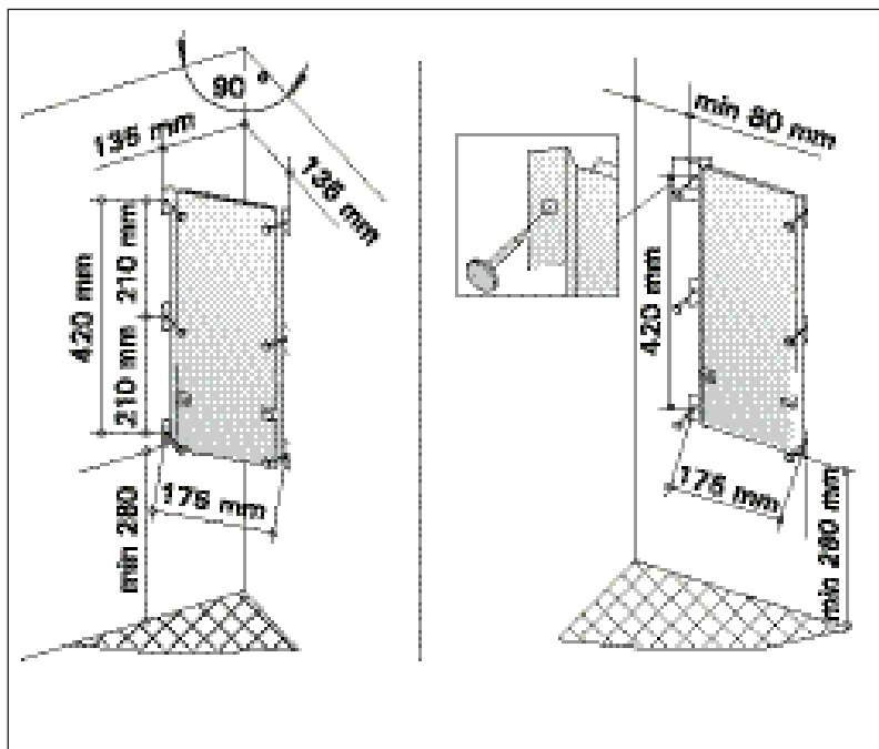
Kuva 7. Kiukaan asennustelineen paikka
