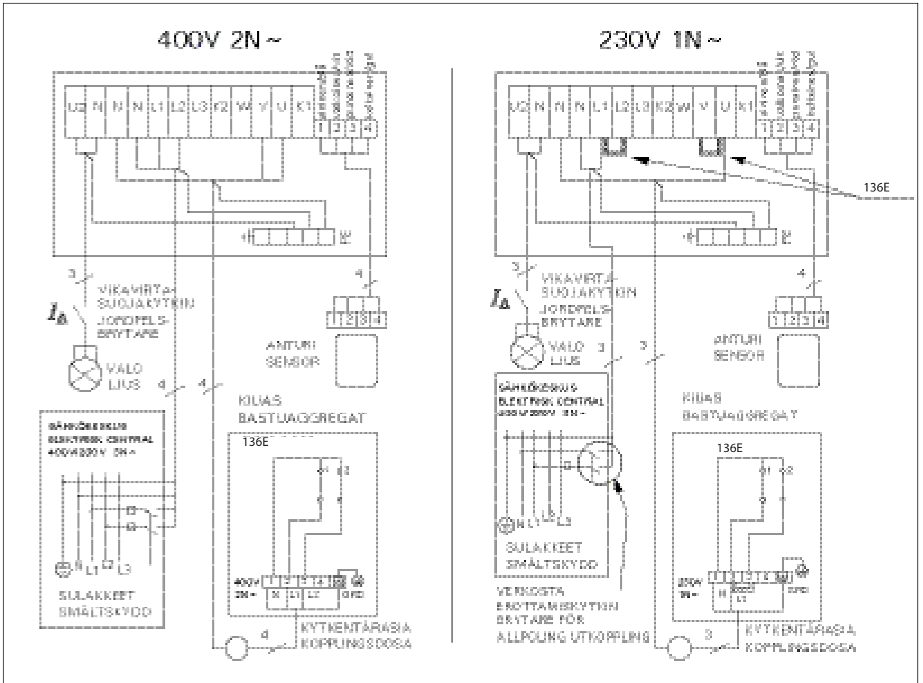
Kuva 12. Ohjaukeskuksen ja kiukaan sähkökytkennät (136E) Bild 12. Elininstallationer av styrcentral och aggregat (136E)
